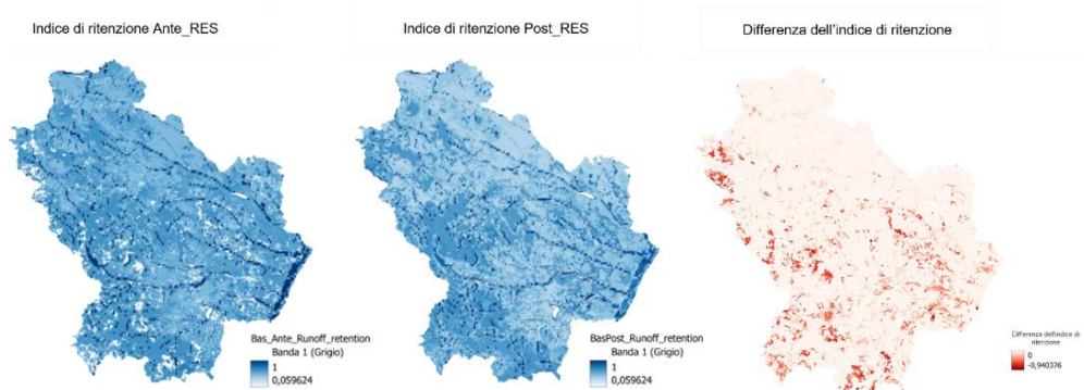
Figura 200. A sinistra le mappe dell'indice di ritenzione del deflusso superficiale. Visualizzazione comparativa delle condizioni pre-RES (sinistra) e post-RES (destra) mediante scale cromatiche identiche. Lo schiarimento delle tonalità in prossimità dei cluster RES indica una ridotta capacità di ritenzione idrica. A destra la mappa delle differenze dell'indice di Ritenzione del Deflusso
